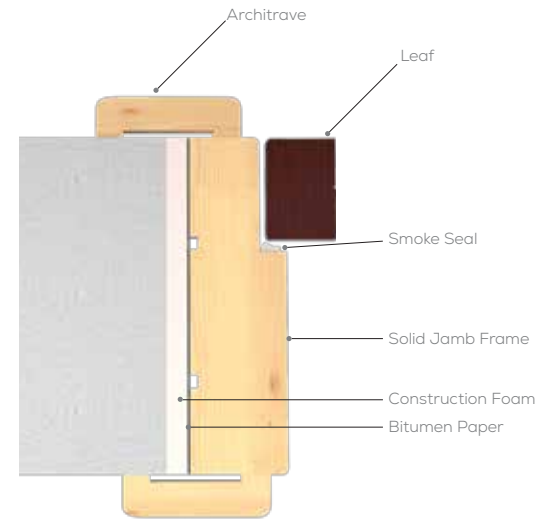
SOLID JAMB FRAME
